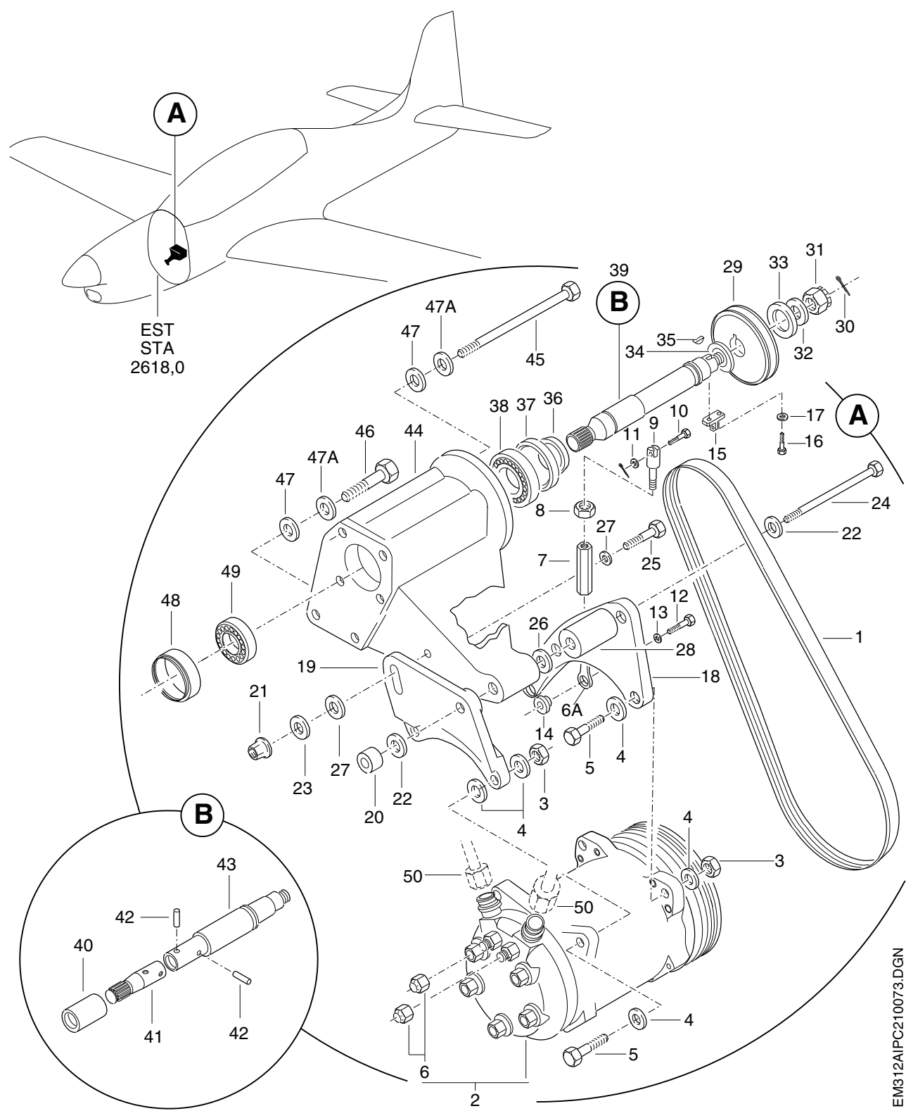
FIGURA 06. INSTALACAO DO COMPRESSOR FIGURE 06. COMPRESSOR INSTL
