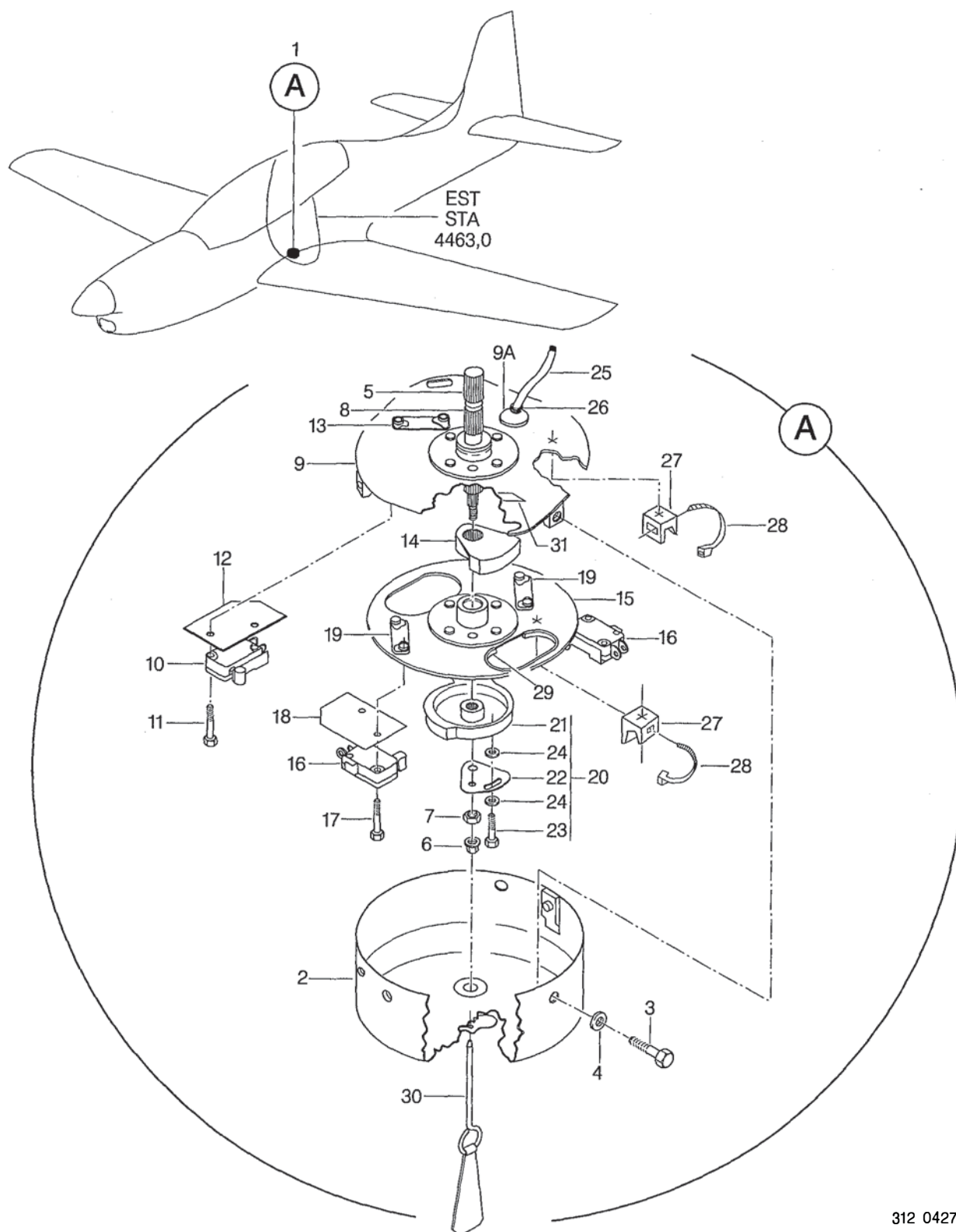
FIGURA 02. UNIDADE DE CONTROLE DE POSICAO DO FLAPE FIGURE 02. FLAP POSITION CONTROL UNIT
