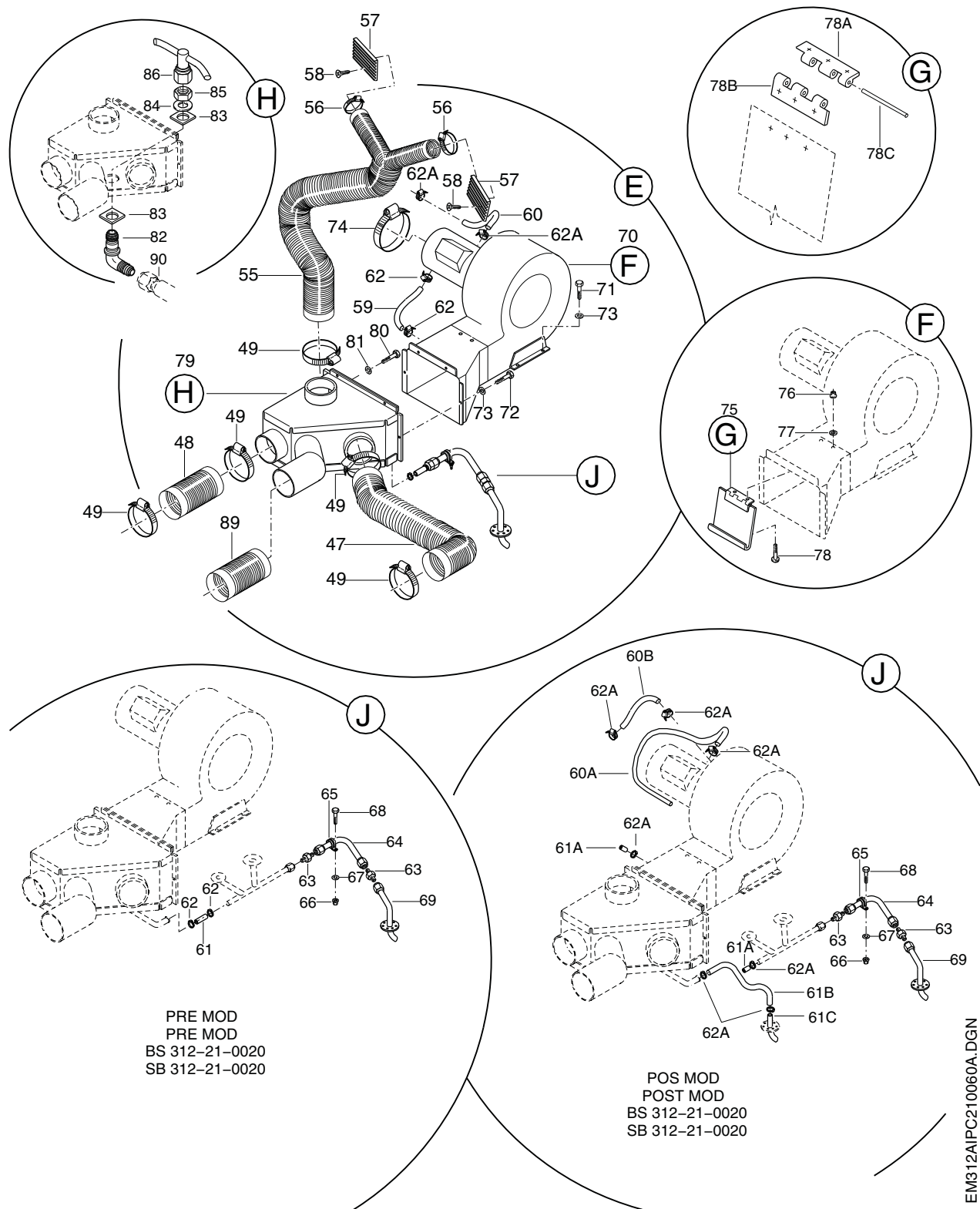
FIGURA 04. DISTRIBUIÇÃO DE AR CONDICIONADO INSTL (FOLHA 3 DE 3) FIGURE 04. AIR CONDITIONING DISTRIBUTION INSTL (SHEET 3 OF 3)
