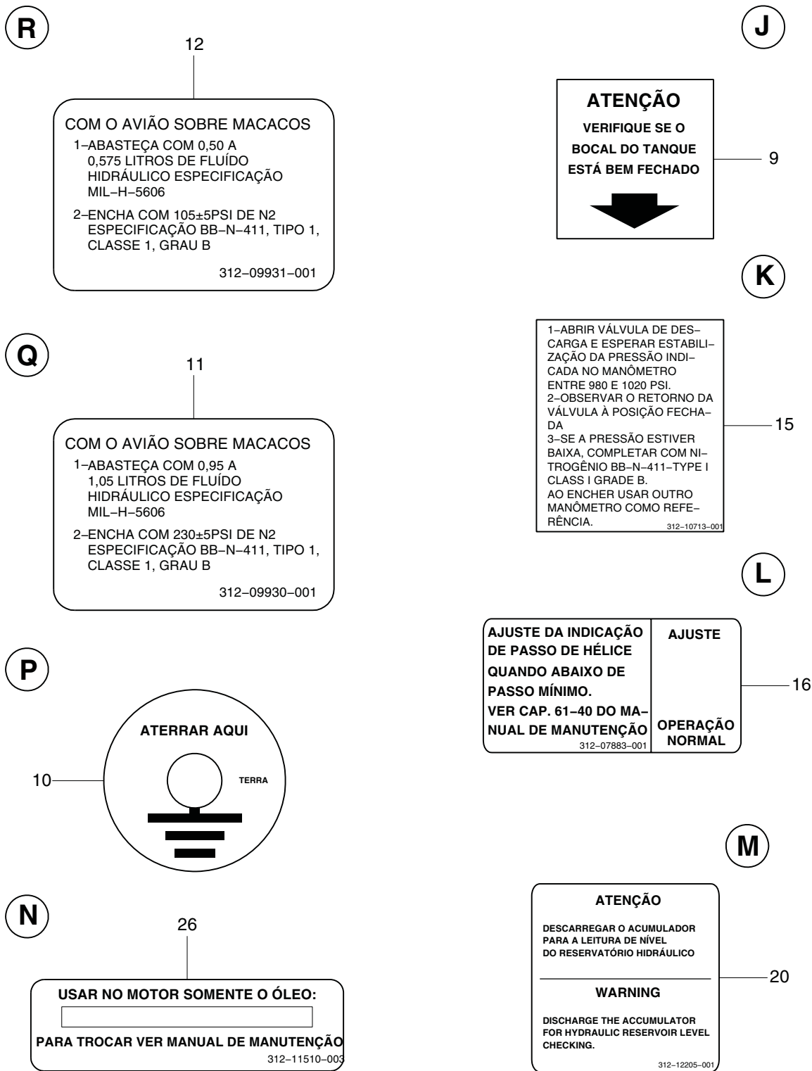
FIGURA 01. INSCRICOES E MARCACOES EXTERNAS INSTL (FOLHA 4 DE 5) FIGURE 01. EXTERIOR PLACARDS & MARKINGS INSTL (SHEET 4 OF 5)
