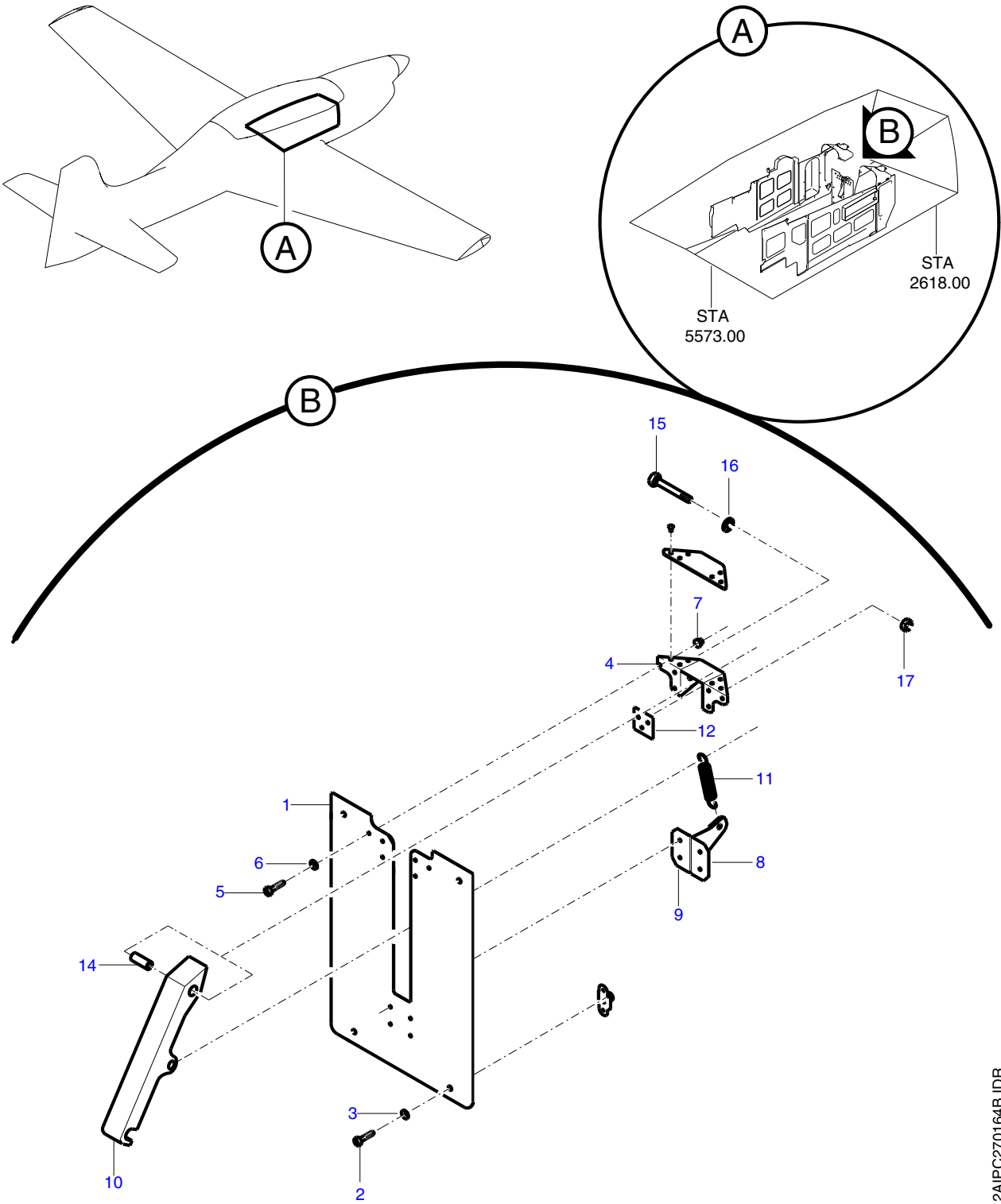
FIGURA 01. SISTEMA DE TRAVA COMANDO DE SOLO, INSTL FIGURE 01. GUST LOCK SYSTEM, INST
