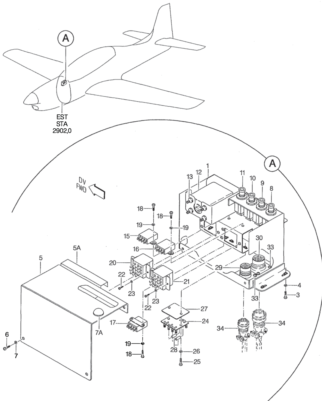
FIGURA 01. CAIXA DE RELES AC INSTL FIGURE 01. AC RELAY BOX INSTL
