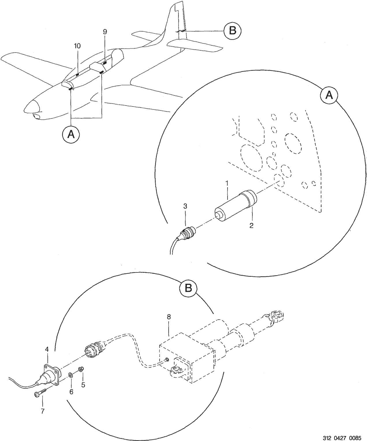
FIGURA 01. SISTEMA DE INDICACAO INSTL, COMPENSADOR DO LEME DE DIRECAO FIGURE 01. POSITION INDICATING SYSTEM INSTL, RUDDER TRIM TAB
