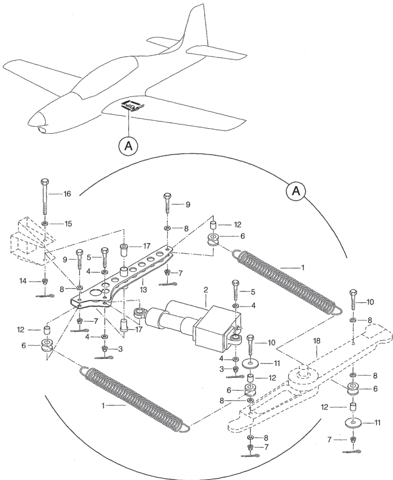
FIGURA 01. COMANDO DO COMPENSADOR INSTL, AILERON FIGURE 01. AILERON TRIM TAB CONTROL INSTL
