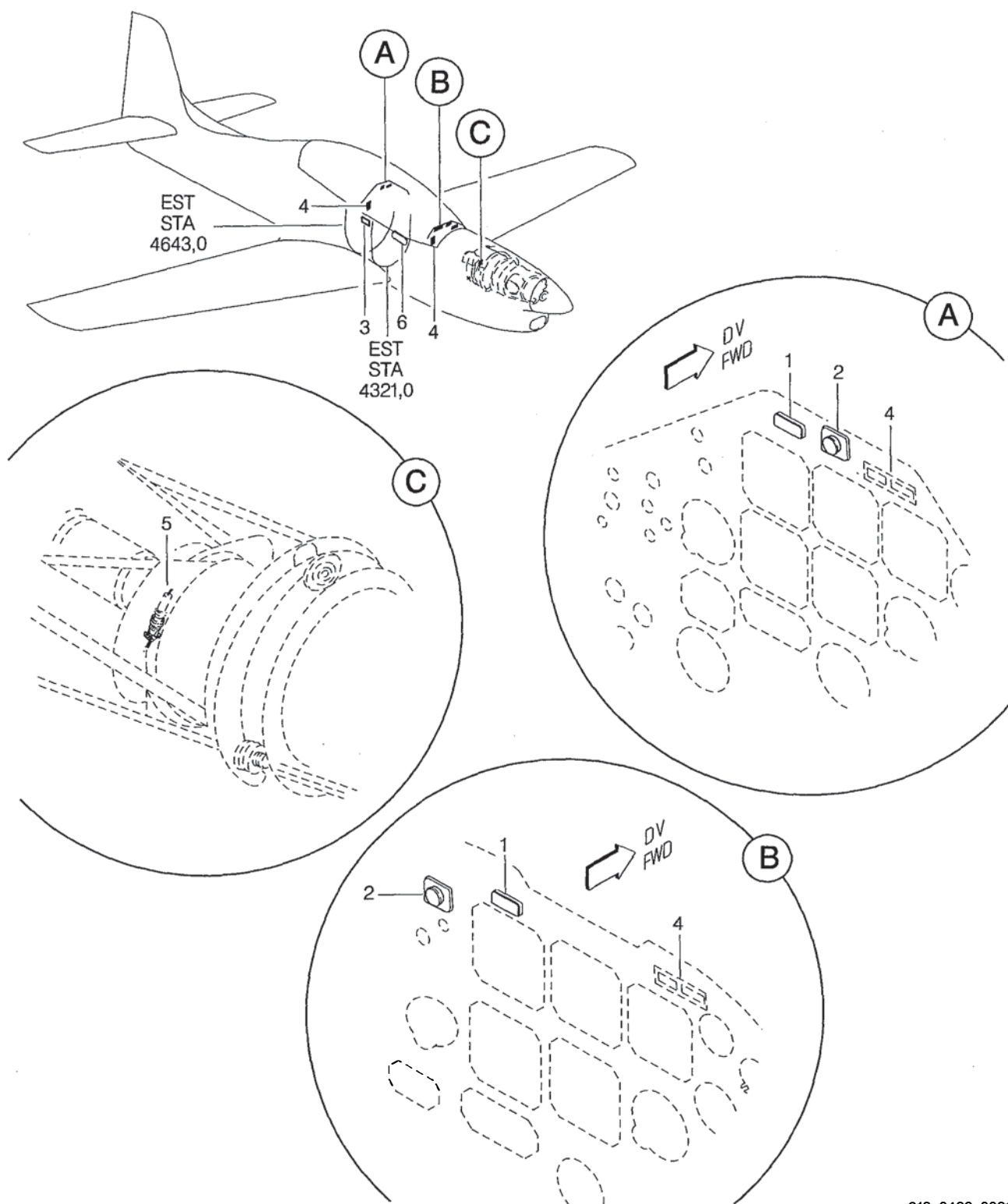
FIGURA 02. SISTEMA DE INDICACAO INSTL, ALARME DE FOGO FIGURE 02. FIRE ALARM INDICATING SYSTEM INSTL
