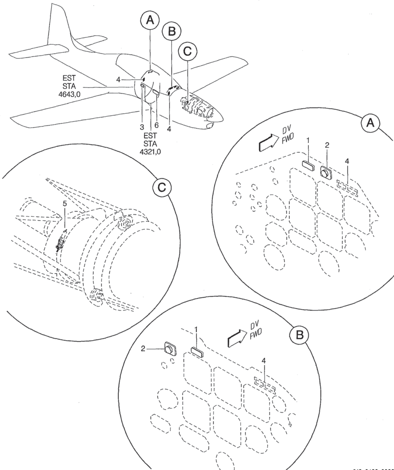
FIGURA 03. SISTEMA DE INDICACAO INSTL, ALARME DE FOGO FIGURE 03. FIRE ALARM INDICATING SYSTEM INSTL
