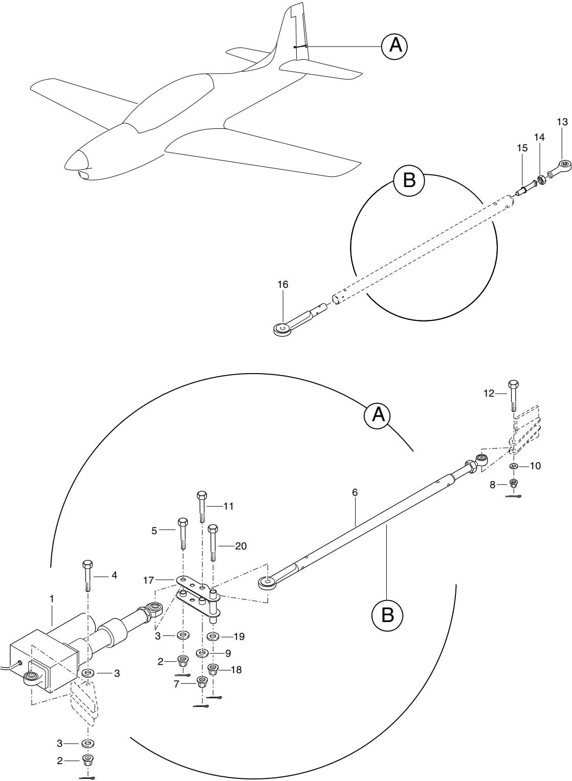
FIGURA 01. SISTEMA DE ATUACAO DO TAB DO LEME INSTL FIGURE 01. RUDDER TRIM TAB ACTUATING SYSTEM INSTL
