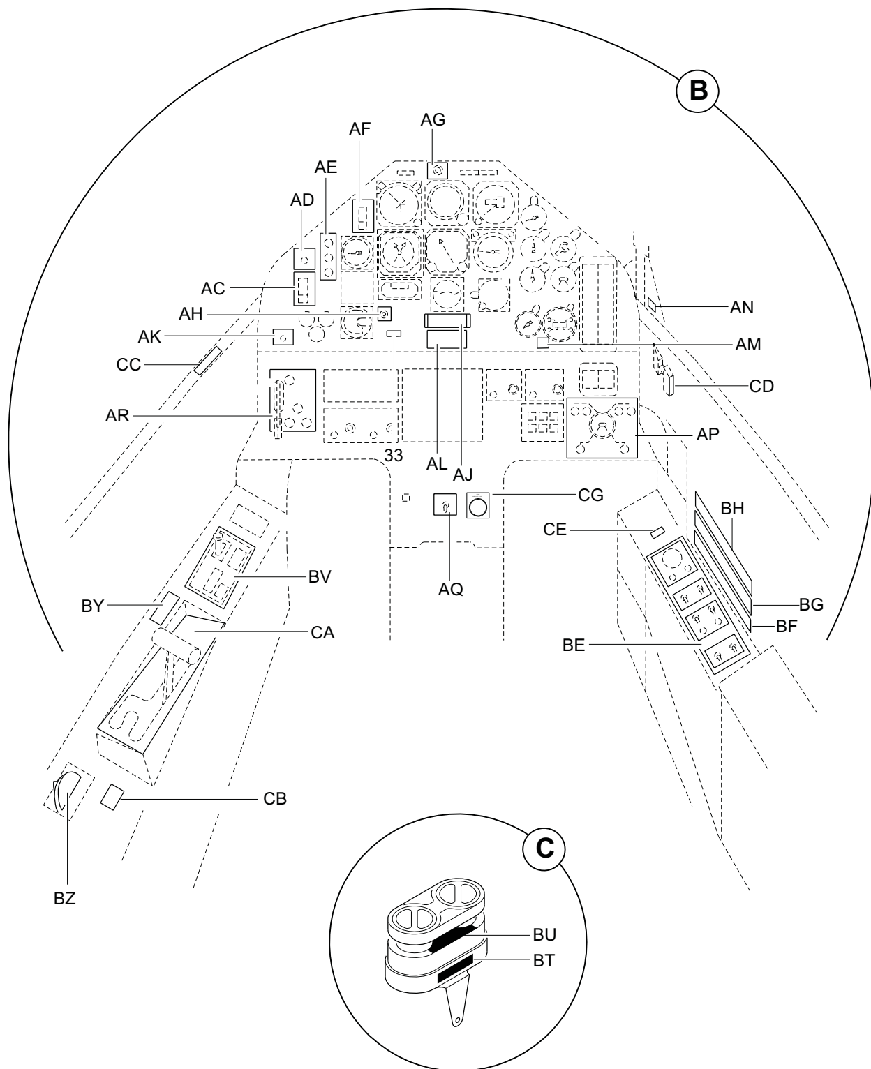
FIGURA 01. INSCRIÇÕES E MARCAÇÕES INTERNAS INSTL (FOLHA 2 DE 15) FIGURE 01. INTERIOR PLACARDS & MARKINGS INSTL (SHEET 2 OF 15)
