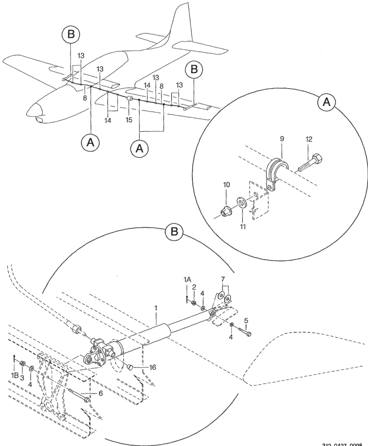
FIGURA 01. ATUADORES DOS FLAPES INSTL FIGURE 01. FLAP LINEAR ACTUATORS INSTL
