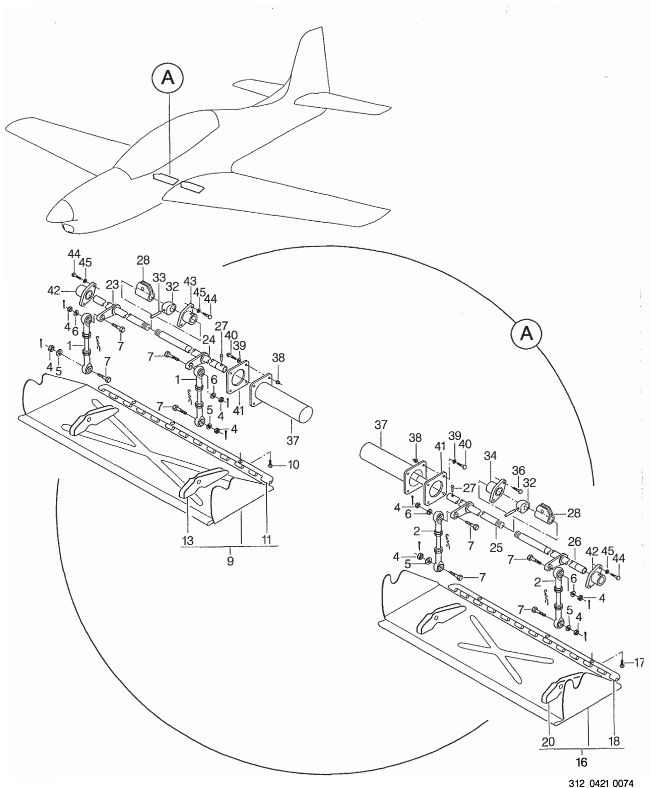
FIGURA 10. TOMADAS DE AR DOS CONDENSADORES INSTL FIGURE 10. CONDENSER AIR SCOOPS INSTL
