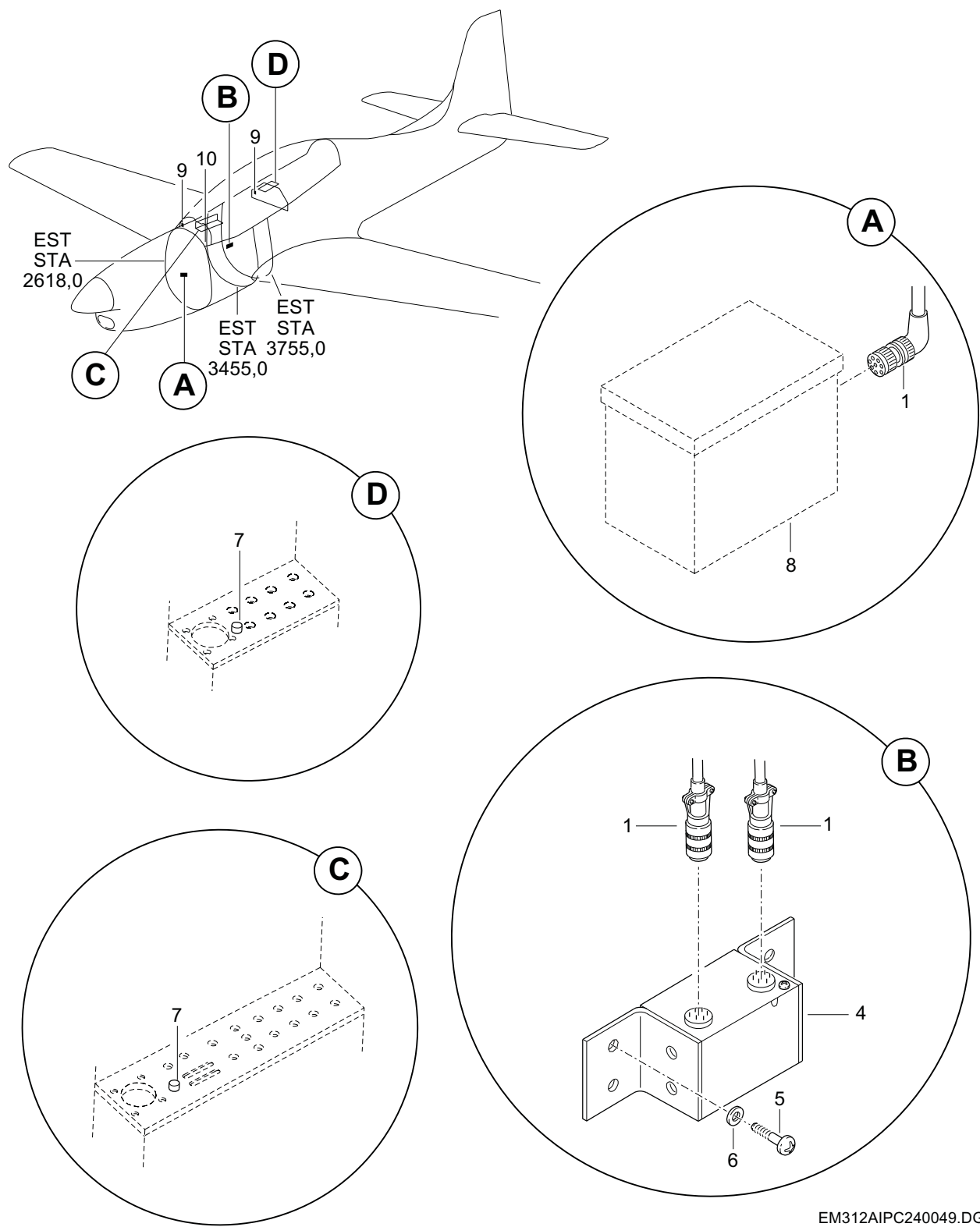
FIGURA 01. INDICACAO DE TEMPERATURA DA BATERIA INSTL FIGURE 01. BATTERY TEMP MONITORING SYSTEM INSTL
