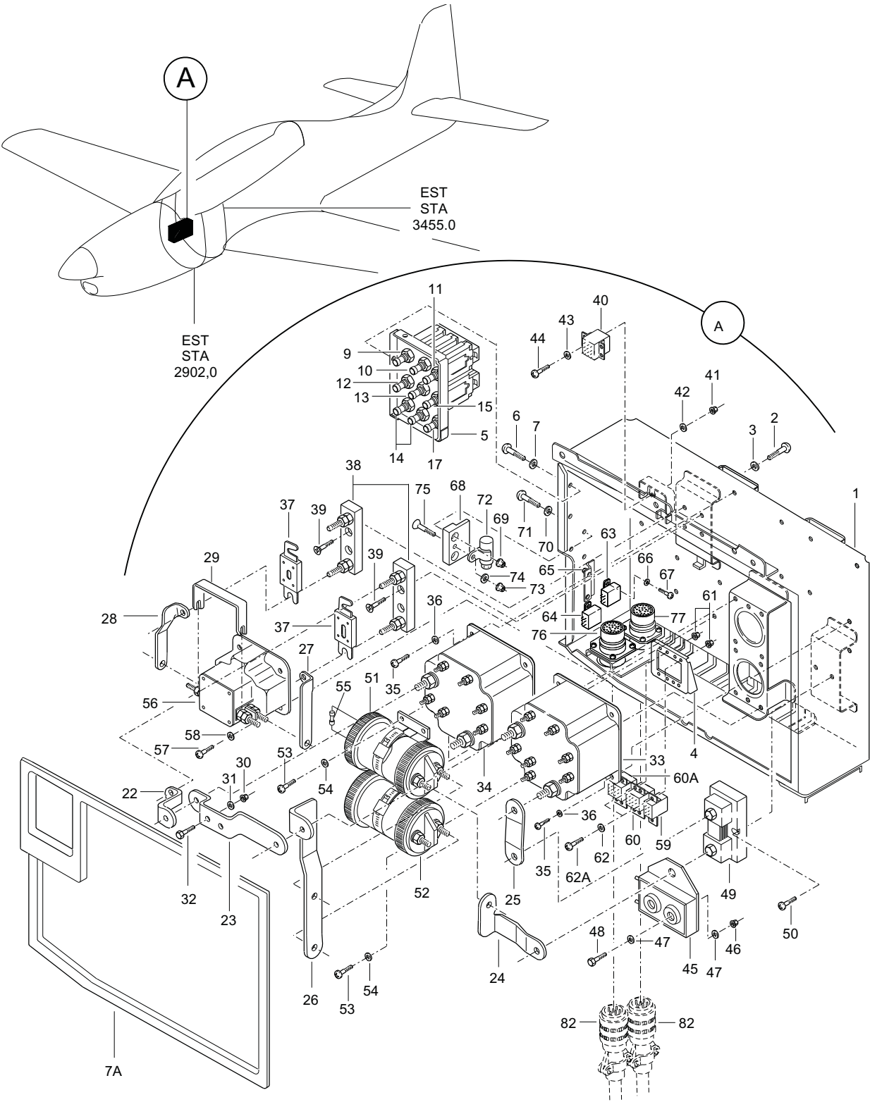
FIGURA 01.CAIXA DE RELES DC INSTL FIGURE 01.DC RELAY BOX INST
