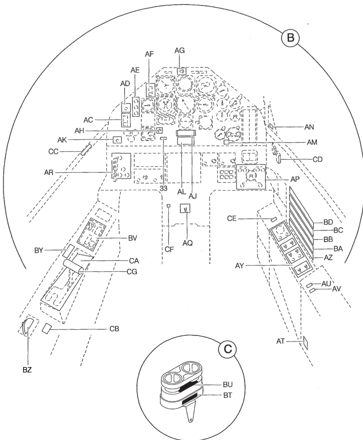
FIGURA 05. INSCRIÇÕES E MARCAÇÕES INTERNAS INSTL (FOLHA 2 DE 12) FIGURE 05. INTERIOR PLACARDS & MARKINGS INSTL (SHEET 2 OF 12)
