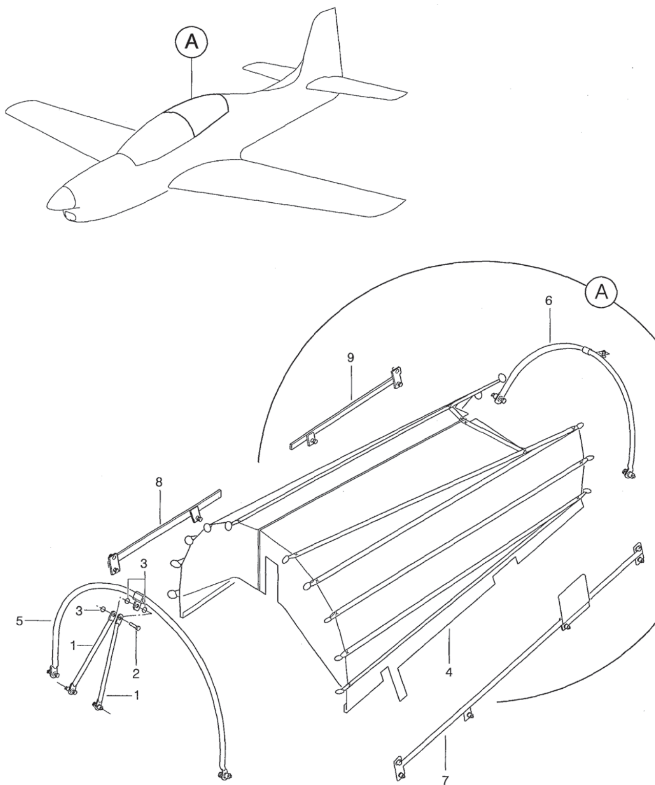
FIGURA 07. CAPOTA P/ VOO POR INSTRUMENTO INSTL FIGURE 07. BLIND INSTRUMENT FLYING HOOD INSTL
