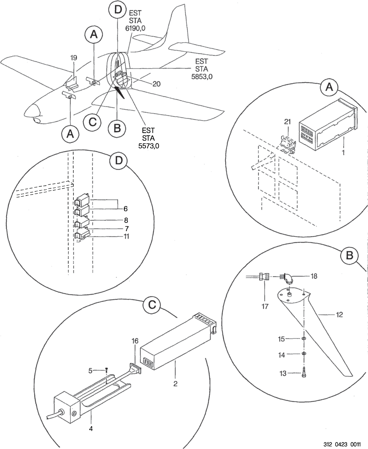
FIGURA 01. SISTEMA VHF1 INSTL FIGURE 01. VHF1 SYSTEM INSTL
