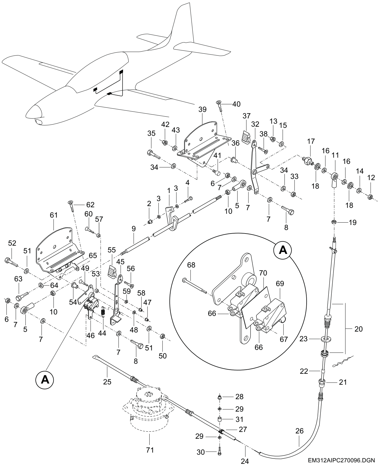
FIGURA 01. SISTEMA DE COMANDO INSTL, FLAPES FIGURE 01. CONTR OL SYSTEM INSTL, FLAP
