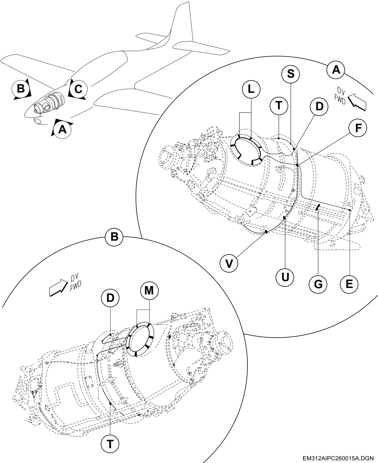
FIGURA 01. SISTEMA DE DETECAO DE FOGO INSTL, MOTOR (FOLHA 1 DE 6) FIGURE 01. FIRE DETECTION SYSTEM INSTL, ENGINE (SHEET 1 OF 6)
