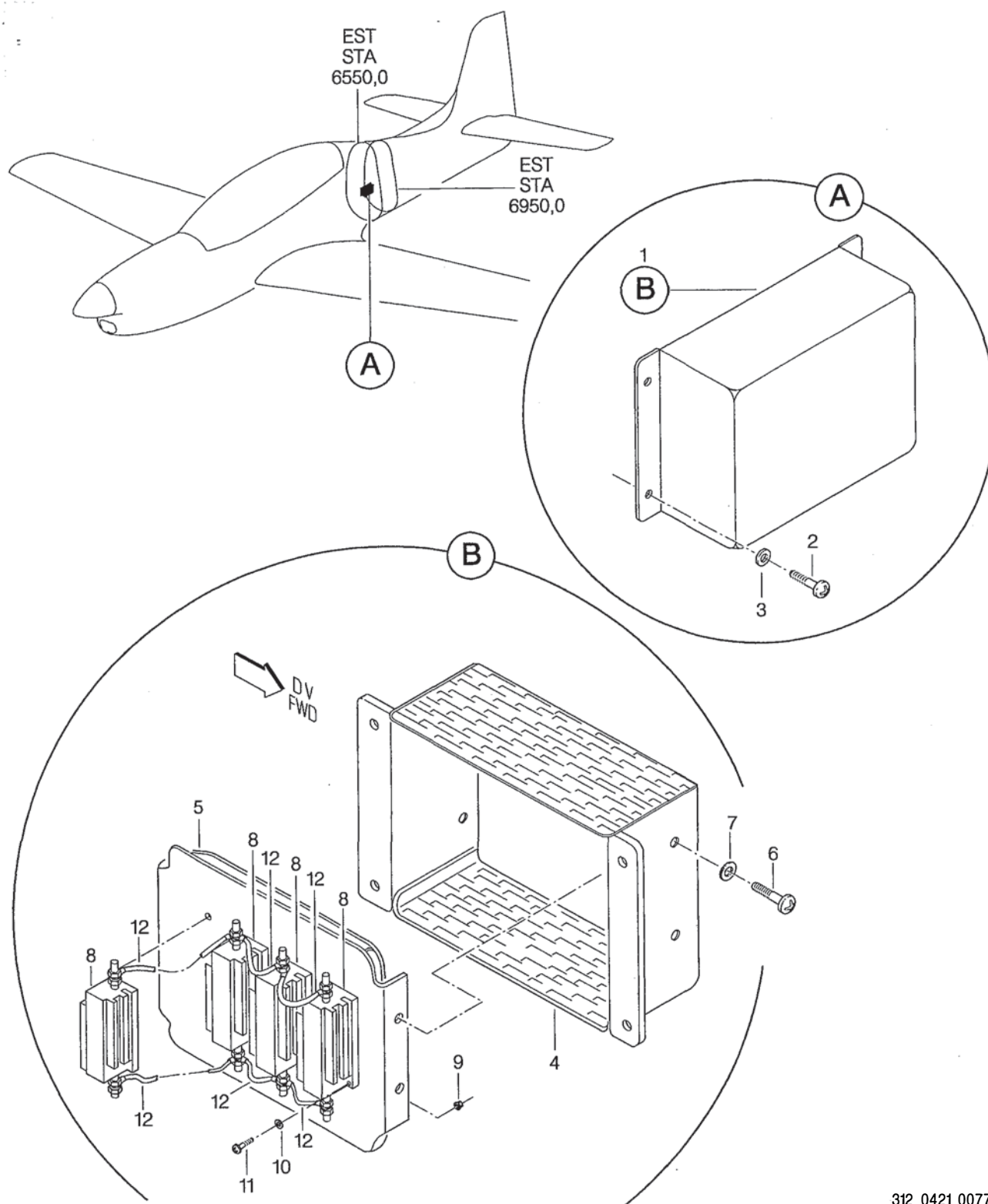
FIGURA 05. CAIXA DE RESISTORES INSTL FIGURE 05. RESISTORS BOX INSTL
