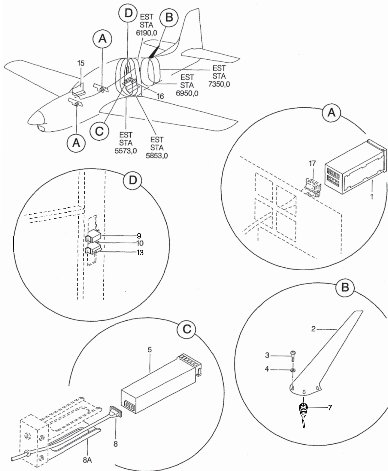
FIGURA 01. SISTEMA VHF2 INSTL FIGURE 01. VHF2 SYSTEM INSTL
