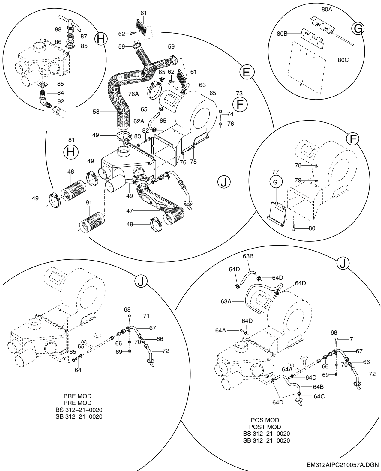
FIGURA 03. DISTRIBUIÇÃO DE AR CONDICIONADO INSTL (FOLHA 3 DE 3) FIGURE 03.AIR CONDIT/ONING DISTRIBUTION INSTL (SHEET 3 OF 3)
